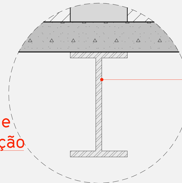
Detalhe viga metálica corte
