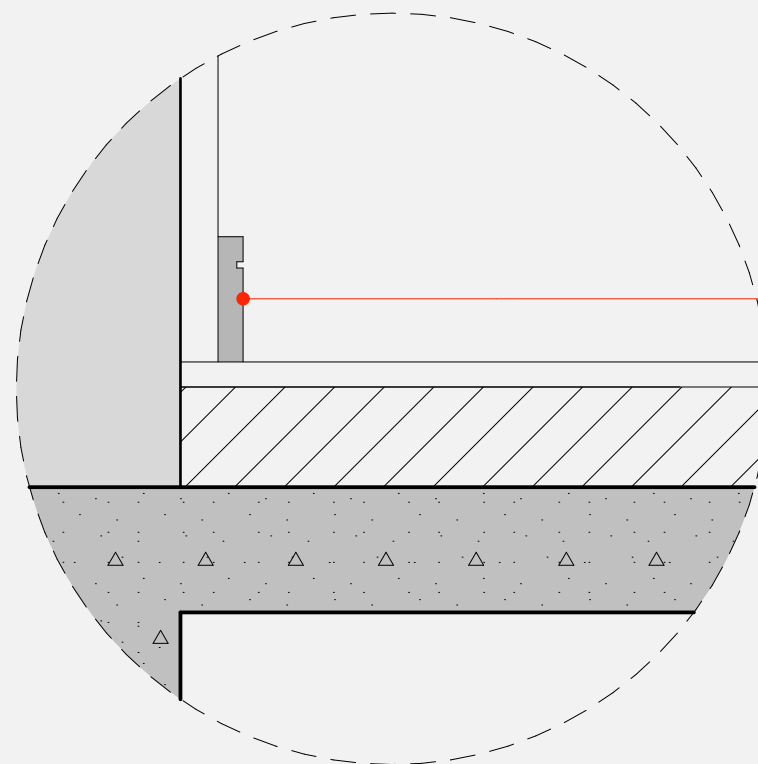
Detalhe rodapé corte
