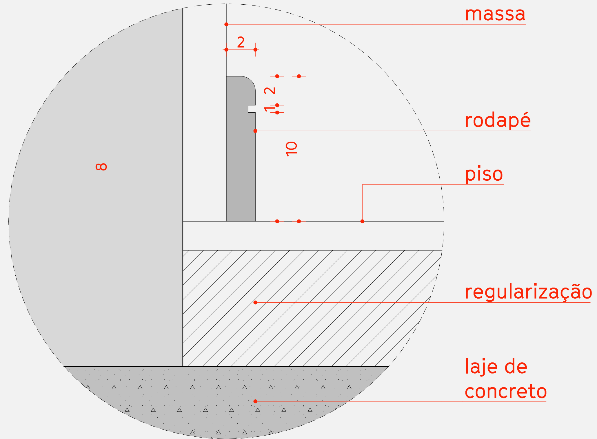
Detalhe rodapé corte
